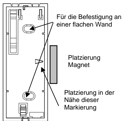
FIG. 2 - Befestigung
